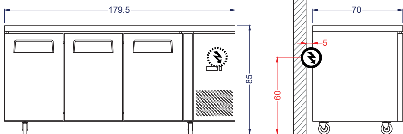
Vista Izquierda
